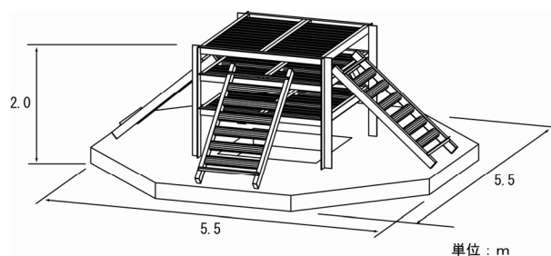
図-2 貝殻増殖礁
